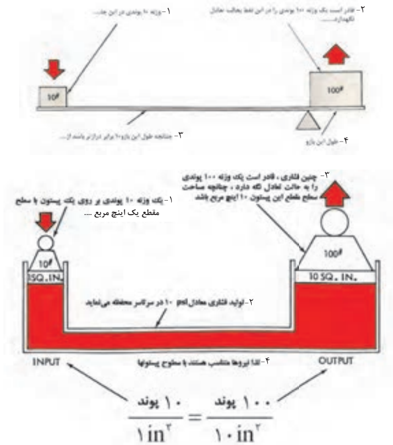
شکل ۱۴-۱- تعادل هیدرولیکی
